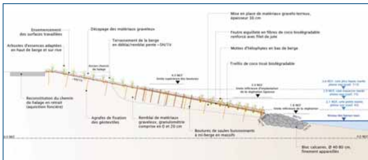
Figure 67 : Exemple de profil semi-végétalisé qui illustre cette séquence mixte : - protection minérale - héliophytes - saulaie (ligneux à bois tendre) - ligneux à bois dur -, réalisé en berge d'estuaire de Seine, avec de très fortes contraintes de battillage et de marée. ≍
