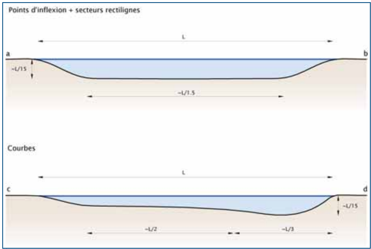
↑ Figure 95 : Exemple de profils en travers (voir le paragraphe précédent pour l'implantation des profils). ≡
