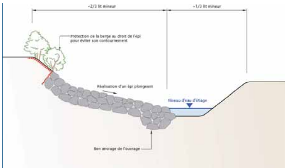
↑ Figure 9 : Schéma « type » d'un épi plongeant en blocs (figure Biotec). ≡
