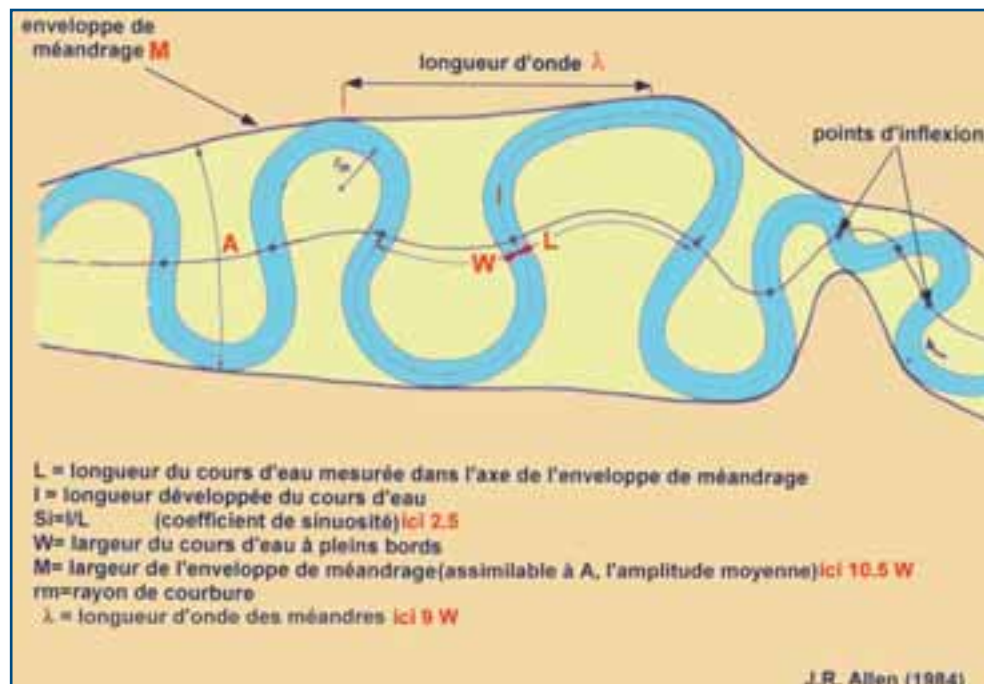
↑ Figure 88 : Mesures morphométriques sur un cours d'eau sinueux. Nota : la largeur « à pleins bords » [sur cette figure « W »] d'un cours d'eau se mesure au droit des points d'inflexion où le profil en travers est le plus symétrique (d'après J.-R. Allen, 1984). 🌊
