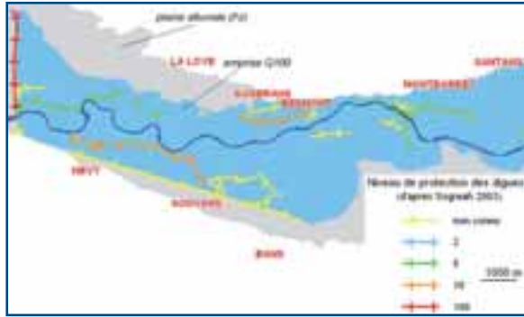
↑ Figure 78 : Exemple d'informations concernant le réseau de digues (positionnement, fréquence de submersion) (source : Malavoi, Safège, 2006). ≍
