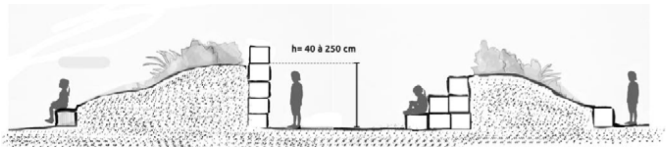
Typologie avec soutènement : assises, gradins et mur © CAUE de Paris
