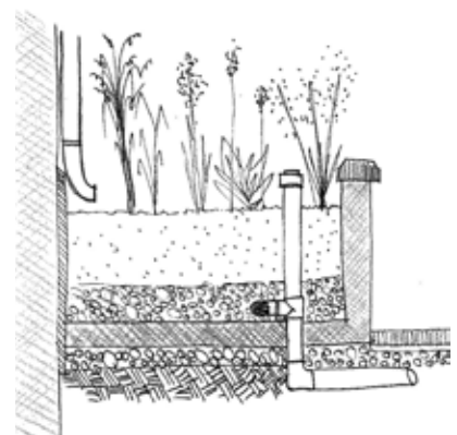
Jardinière réservoir © CAUE de Paris
